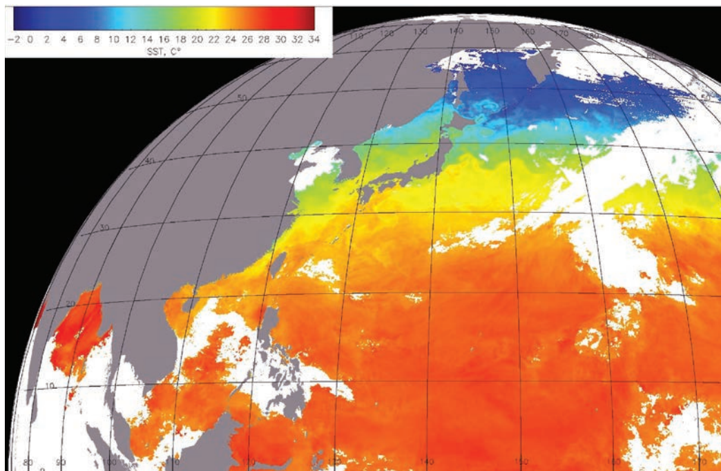
Рис. 1. Глобальная композитная карта температуры поверхности воды по данным КА «MTSAT-1R/2»
