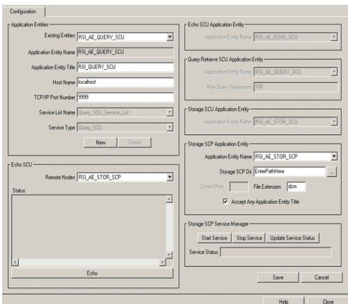
Рис. 2. Графический интерфейс конфигурации DICOM Network Services
